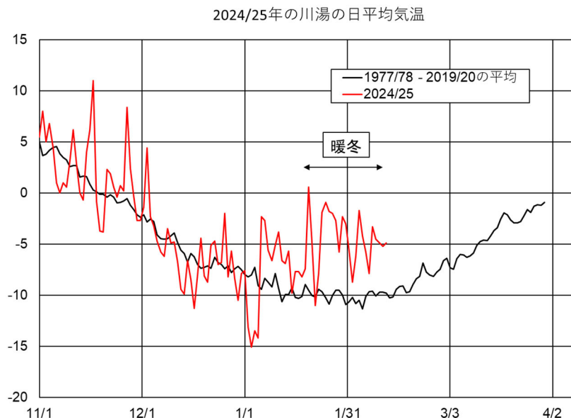
図1 川湯アメダスの日平均気温の推移(暖冬期間を両矢印で示す)。
